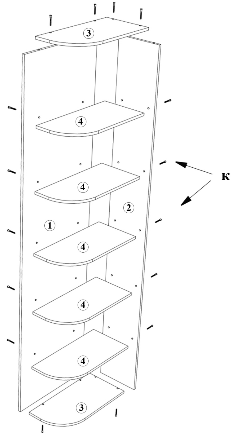
Схема складання консолі
